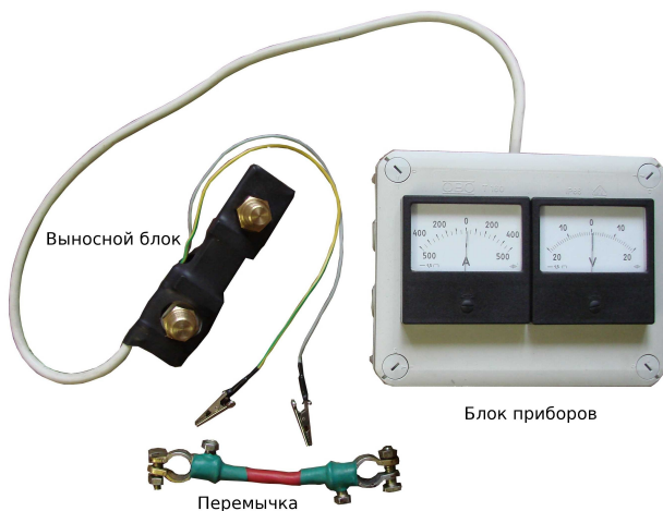
Рисунок 1 - Тестер АСГ
