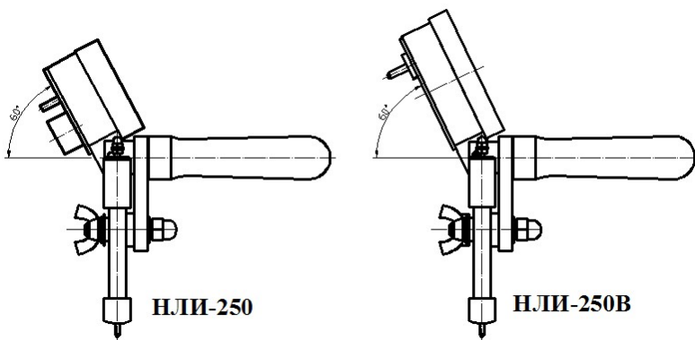
Рисунок 6 – Возможные положения вольтметра нагрузочной вилки НЛИ-250
