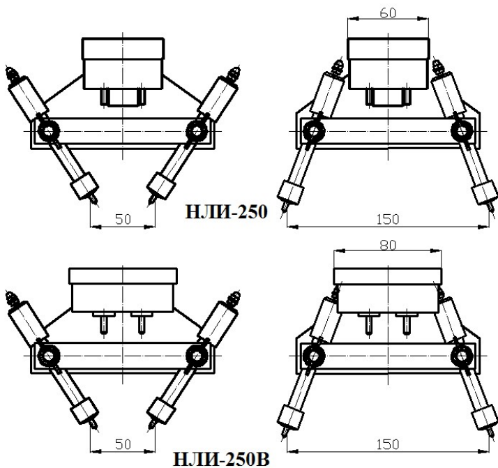
Рисунок 5 – Настройка вилки нагрузочной на размер между выводами аккумулятора.
