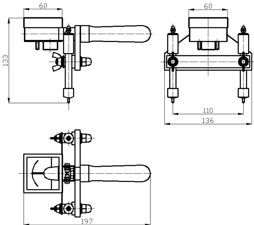
Рисунок 3 – Габаритные размеры вилки нагрузочной НЛИ-250.
