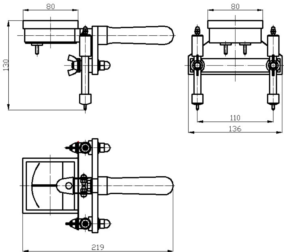
Рисунок 4 – Габаритные размеры вилки нагрузочной НЛИ-250В.
