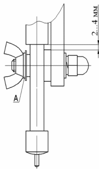
Рисунок 1 - Установка размера 2...4 мм
